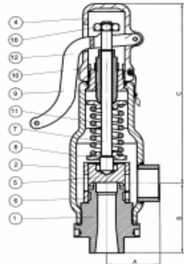
AVEC LEVIER
